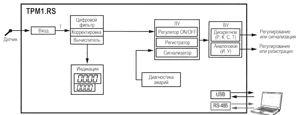
Рисунок 6.1 – Функциональная схема
