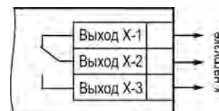
Рисунок 5.22 – Схема подключения нагрузки к ВУ типа «Р»
