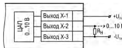
Рисунок 5.29 – Схема подключения нагрузки к ВУ типа «У»
