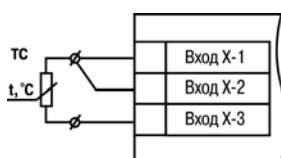
Рисунок 5.16 – Трехпроводная схема подключения ТС
