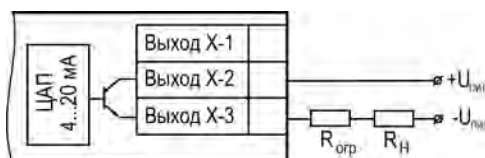
Рисунок 5.28 – Подключение к ВУ типа «И» с ограничивающим резистором
