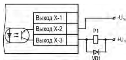
Рисунок 5.23 – Схема подключения нагрузки к ВУ типа «К»
