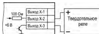
Рисунок 5.24 – Схема подключения нагрузки к ВУ типа «Т»
