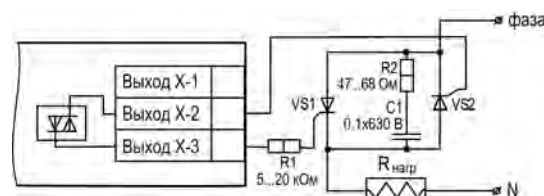
Рисунок 5.26 – Схема встречно-параллельного подключения двух тиристоров к ВУ типа «С»
