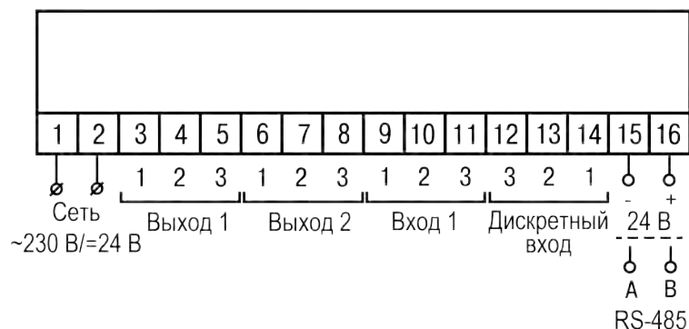
Рисунок 5.4 – Общая схема подключения ТРМ10–Щ1/Щ2
