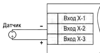
Рисунок 5.19 – Схема подключения активного датчика с выходом в виде напряжения -50...+50 мВ или 0...1 В
