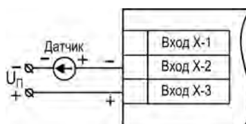
Рисунок 5.21 – Схема подключения пассивного датчика с токовым выходом 0...5 мА или (4)...20 мА
