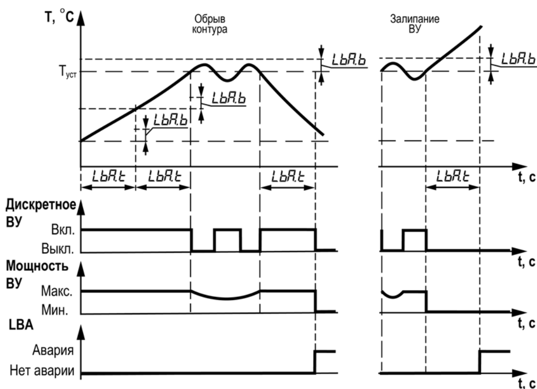
Рисунок 7.5 – Принцип работы диагностики обрыва контура регулирования
