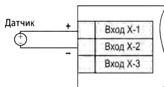
Рисунок 5.20 – Схема подключения активного датчика с выходом в виде напряжения 0...5 В и 0...10 В
