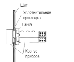
Рисунок 1 – Монтаж прибора
