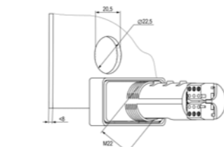
Рисунок 2 – Установочные размеры прибора
