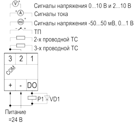
Рисунок 8 – Схема подключения входных сигналов и питания
