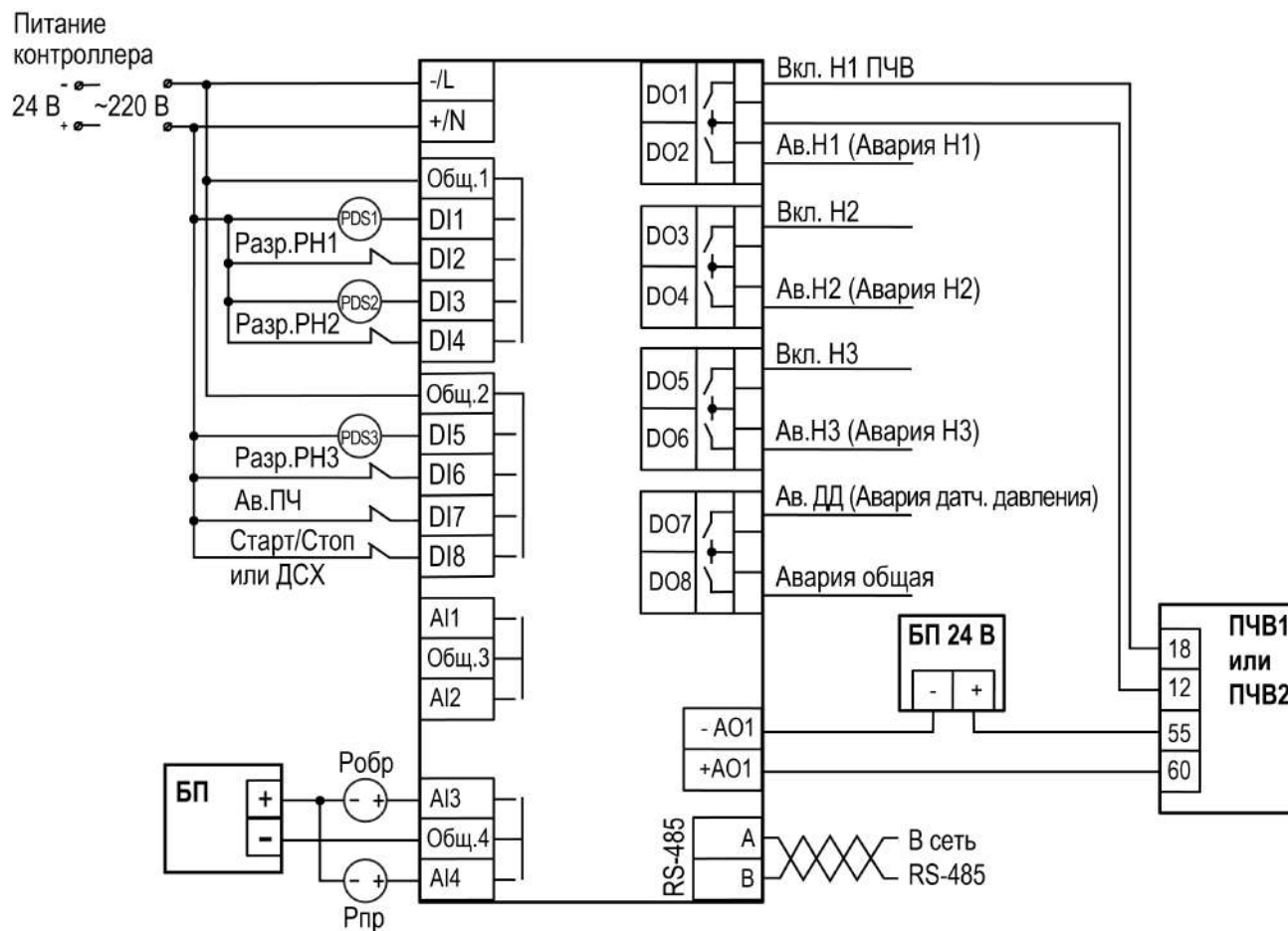
Рисунок 5.5 – Схема подключения СУНА-122.X.05.10
