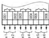
Рисунок 9 – Схема подключения ВЭ типа «Р»
