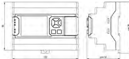
Рисунок 1 – Габаритные размеры прибора
