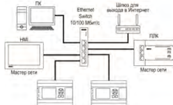
Рисунок 12 – Подключение по схеме «Звезда»
