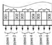
Рисунок 10 – Схема подключения ВЭ типа «Р»
